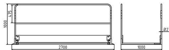
Principskitse for 1,00 x 2,70 m gangbro
