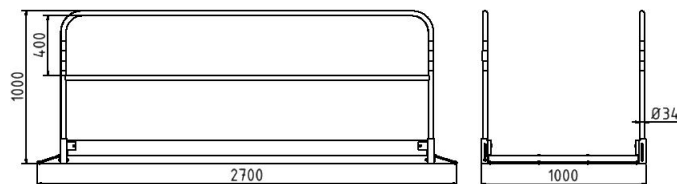
Principskitse for 1,00 x 2,70 m gangbro
